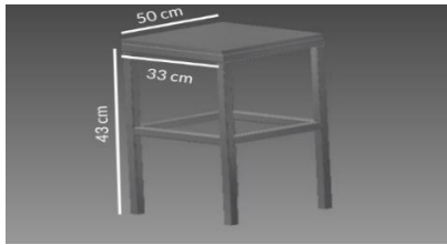
Gambar 7 Desain Rancangan Kursi
