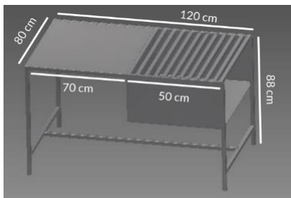
Gambar 8 Desain Rancangan Meja
